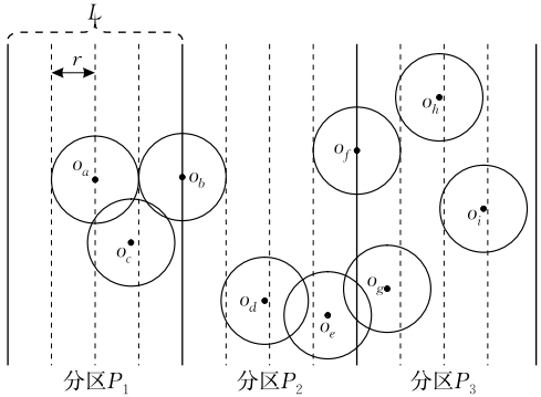
图 4 查询区域按照 L 划分成 3 个分区
